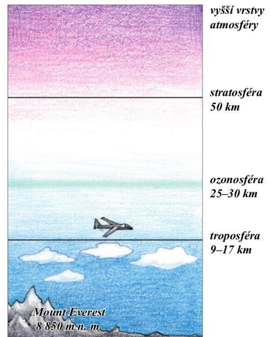
Schéma vrstev atmosféry
